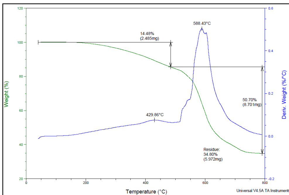
图 2-1 样品 “19121804-3” TGA 曲线
